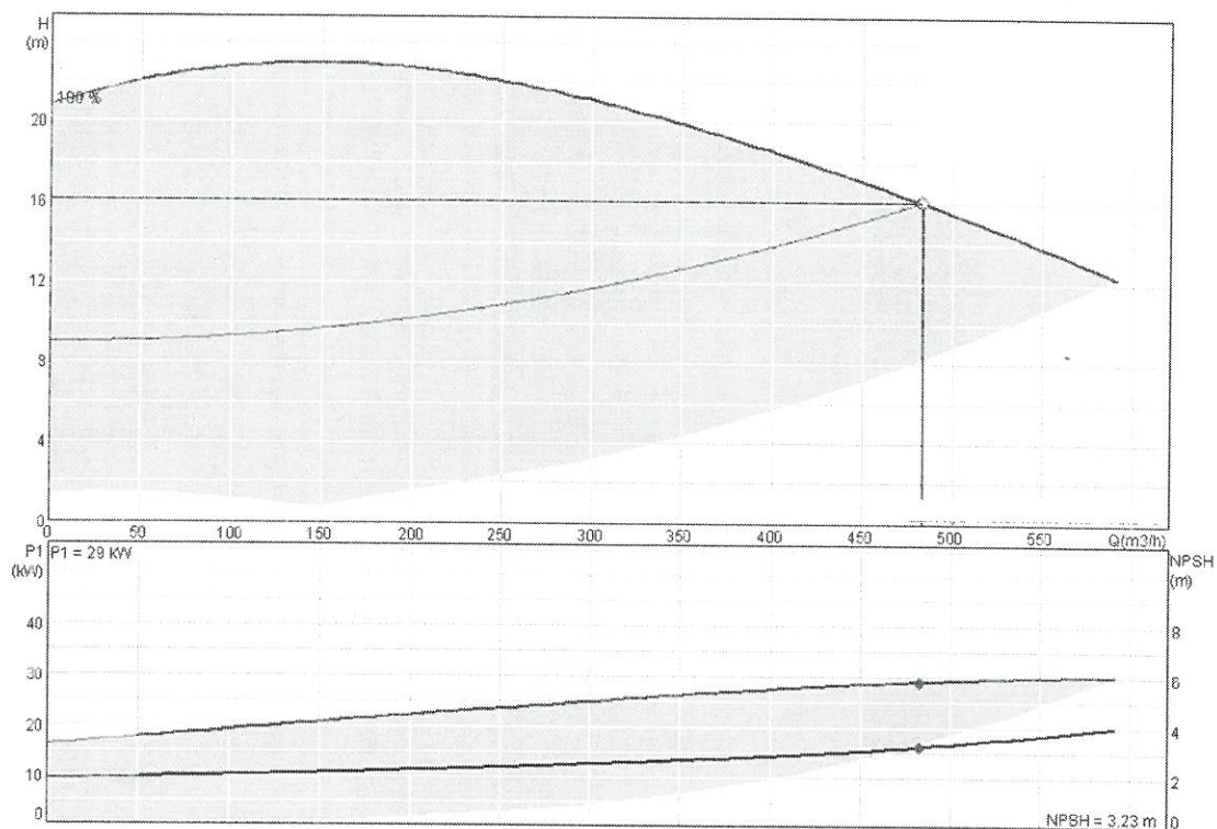
Hálózati jelleggörbe az 1. tétel szivattyújához
