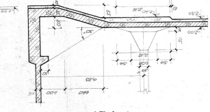
F-METSZET N-1-50
