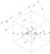
OSZLOPFELFELÜLNÉZET N-1-25
