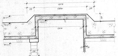
G-METSZET N-1-50
