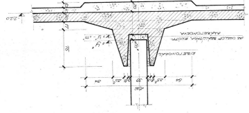
3 JELŰ RÉSZLET N-1-25
